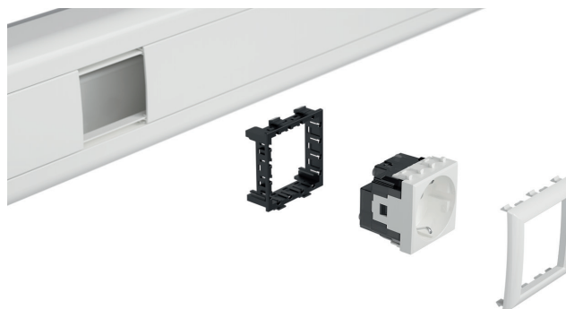
Рабочее место на 2 модуля "Avanti" (1 пост)
